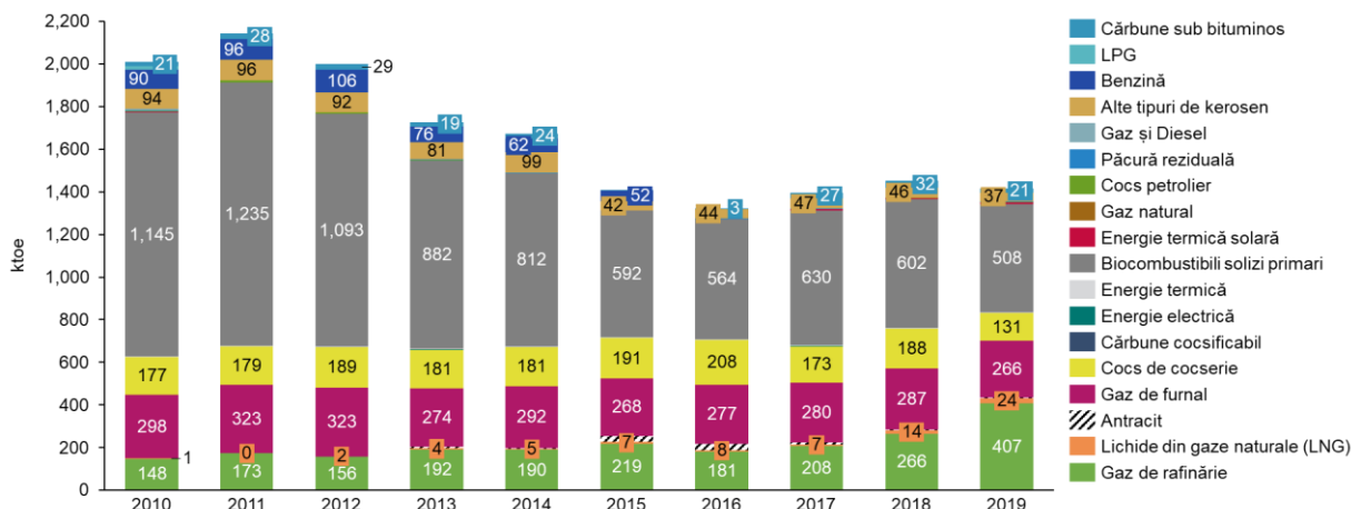
Figura 89. Evoluția consumului final de energie din industria chimică și petrochimică în perioada 2010-2019 (ktoe)
