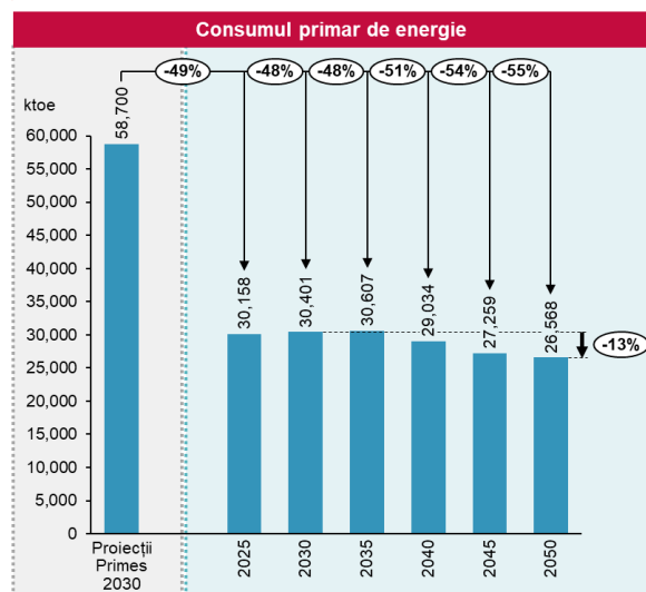
Figura 3. Evoluția consumului primar de energie și țintele intermediare conform scenariului Ro Neutră
