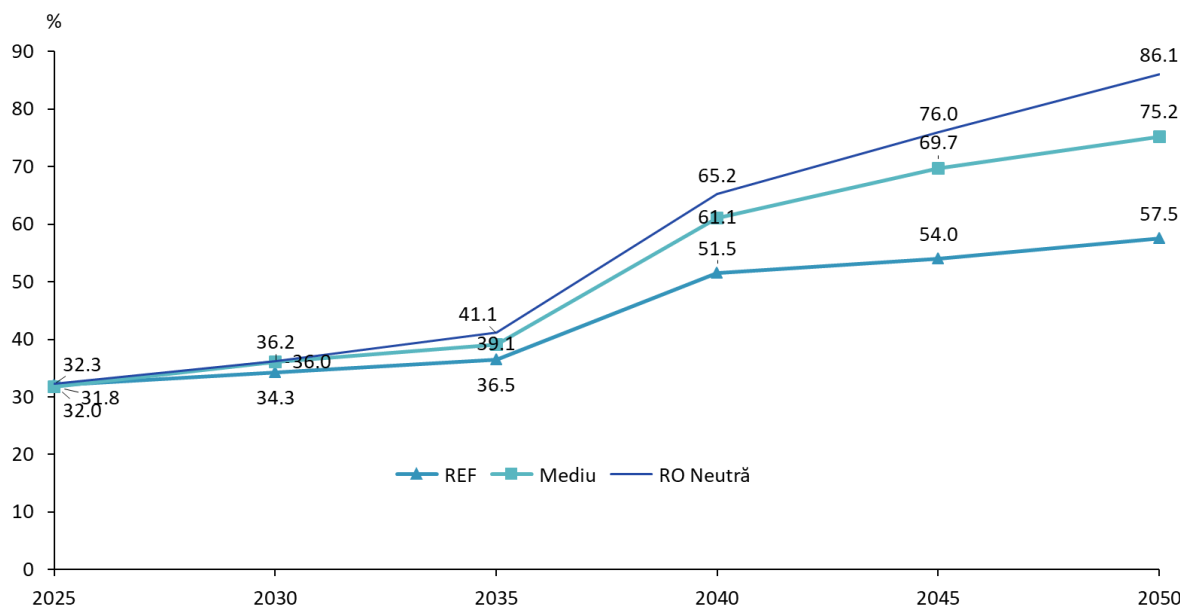
Figura 17. Evoluția ponderii SRE în consumul final brut de energie per tip de combustibil conform celor 3 scenarii analizate: REF, Mediu, RO Neutră
