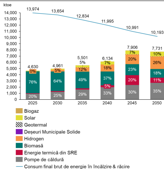
Figura 23. Evoluția SRE per tip de combustibil în consumul final brut de energie în încălzire & răcire
