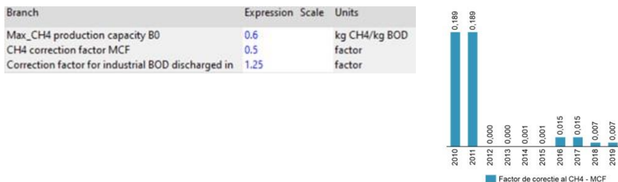
Figura 123. Principalii parametri folosiți pentru modelarea subcategoriilor Neconectat la sisteme de canalizare; Conectat la sisteme de canalizare neconectate la stații de tratare a apelor uzate și fără epurare și Stație de epurare aerobă centralizată
