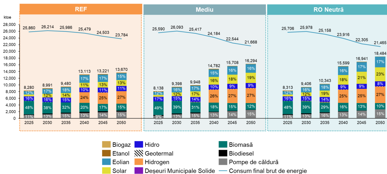
Figura 17. Evoluția ponderii SRE în consumul final brut de energie per tip de combustibil conform celor 3 scenarii analizate: REF, Mediu, RO Neutră
