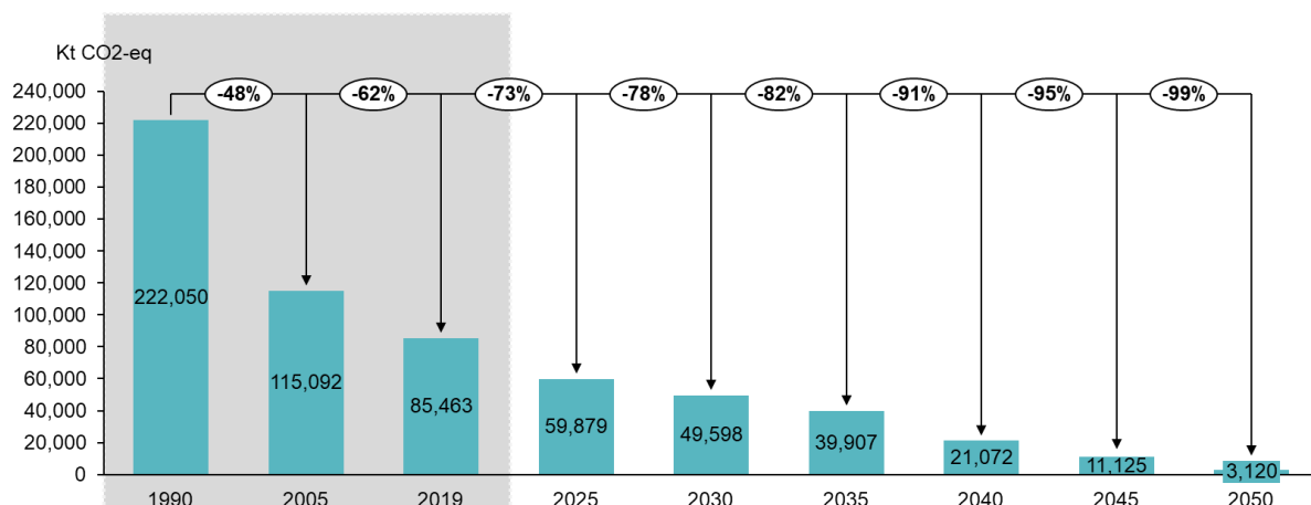
Figura 14. Țintele naționale pentru reducerea emisiilor nete până în 2050 (scenariul RO Neutră)
